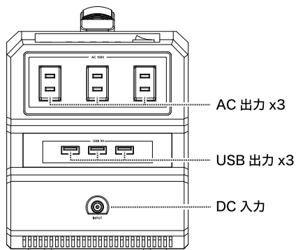
【本体正面】
