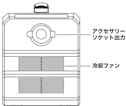
【本体背面】
